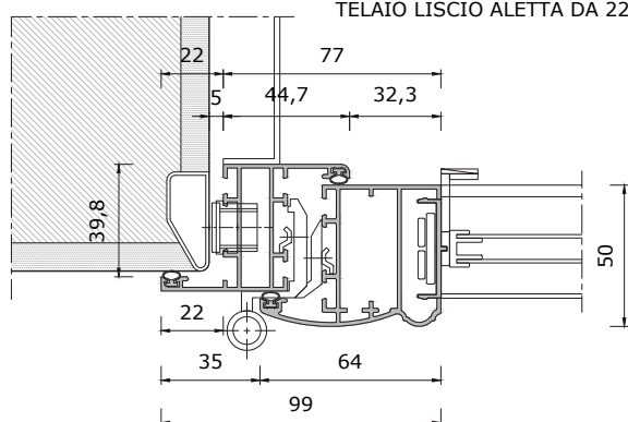
NODO LATERALE TELAIO LISCIO ALETTA DA 22mm
