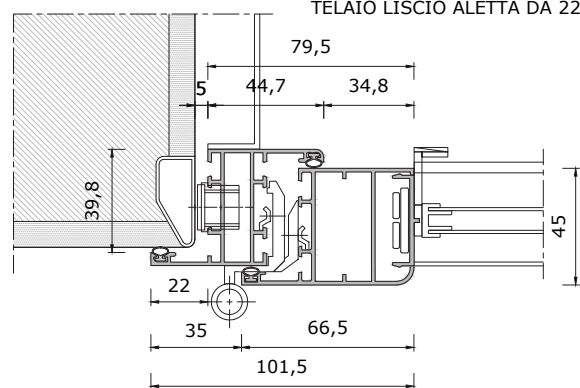
NODO LATERALE TELAIO LISCIO ALETTA DA 22mm
