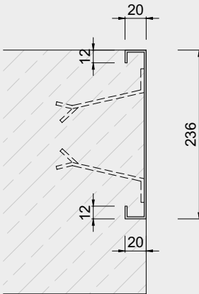
Lamiera a C
