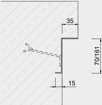
Lamiera a Z
