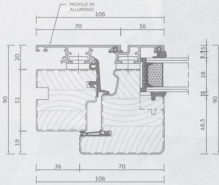
Nodo laterale/superiore
