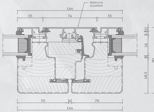
Nodo centrale simmetrico
