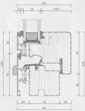
Nodo inferiore finestra
