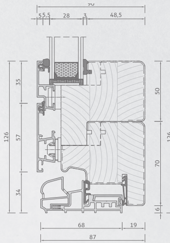
Nodo inferiore portafinestra con vetro unico
